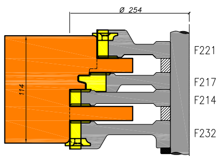
Onderdorpel
