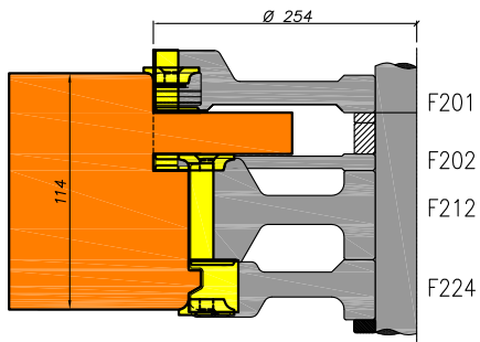
Stijl met scharniersponning
