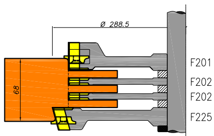
Pennen ramen 3 vlaks
