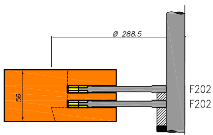
Ramen met kaderdichting onderdorpel
