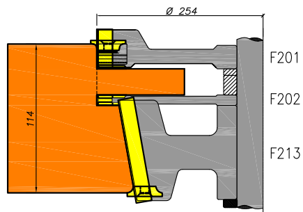
Bovendorpel met waterhol
