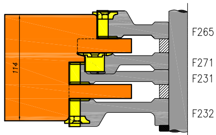
Onderdorpel
