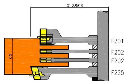
Ramen stijl en bovendorpel met kaderdichting verjongd
