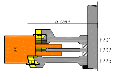
Dubbele pen ramen 56mm
