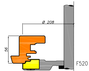
Draaikiep opdek 15mm onderdorpel
