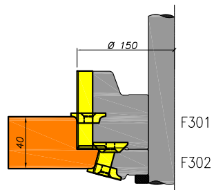
Enkele pen deuren 40/56mm
