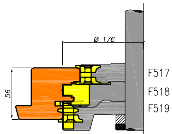
Draaikiep Contura onderdorpel
