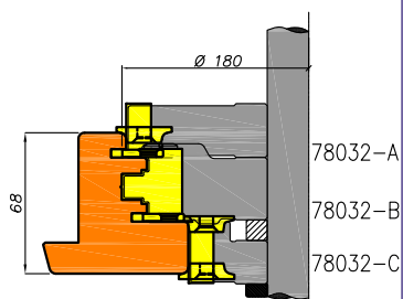
Draaikiep opdek 17mm stomp met dubbelekiërdichting (passive raam)
