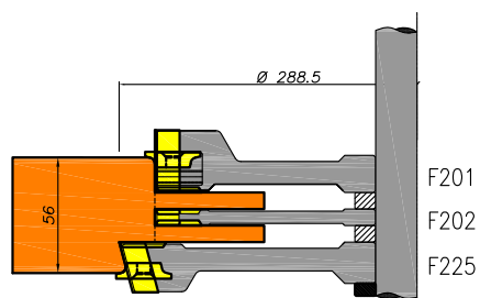
Ramen met kaderdichting en turbohol stijl en bovendorpel
