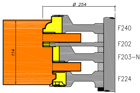
Stijl met scharniersponning
