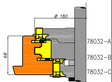
Draaikiep opdek stomp met dubbele kierdichting (passive raam)
