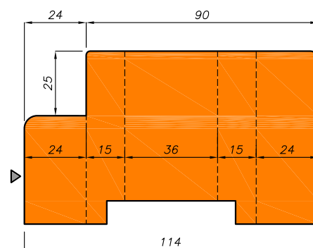
"Opdek"
