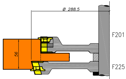
Enkele pen deuren 56mm
