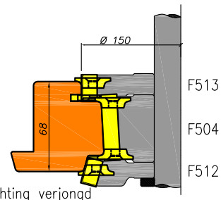
Ramen stijl en bovendorpel met kaderdichting verjongd
