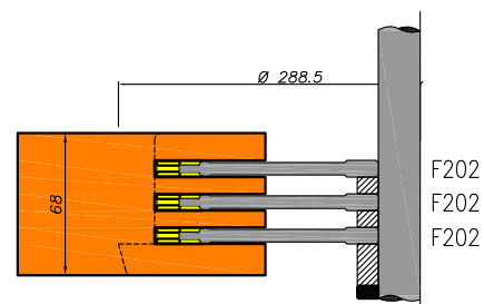
Ramen met kaderdichting onderdorpel
