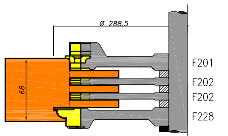
Ramen stijl en bovendorpel met kaderdichting verjongd
