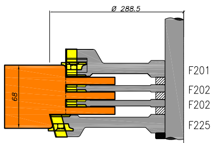
Pennen ramen 3 vlaks
