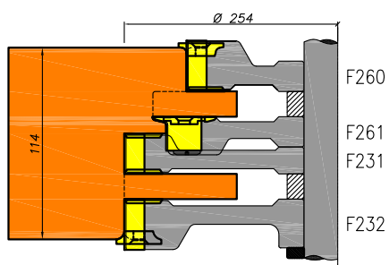
Onderdorpel
