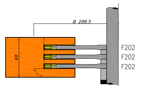
Ramen met kaderdichting onderdorpel
