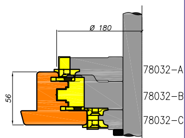
Draaikiep opdek 15mm stomp met dubbelekiërdichting (passive raam)
