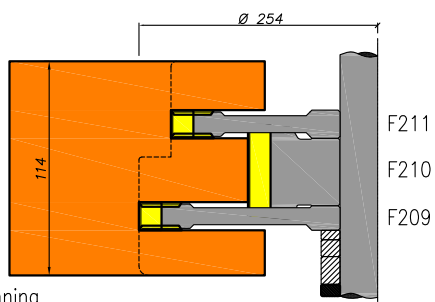
Tussendorpel / kalf
