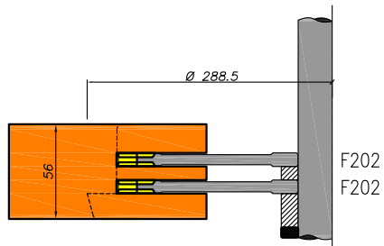
Dubbele pen ramen 56mm
