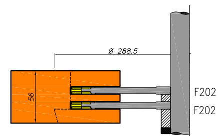
Ramen met kaderdichting en turbohol onderdorpel
