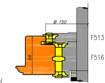
Ramen met kaderdichting onderdorpel
