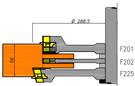
Stompe ramen stijl en bovendorpel verjongd
