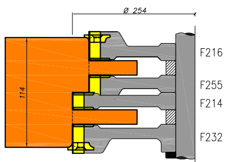
Onderdorpel
