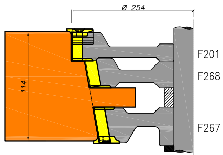
Onderdorpel
