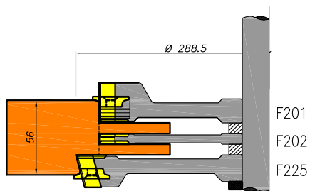
Draaikiep Contura
