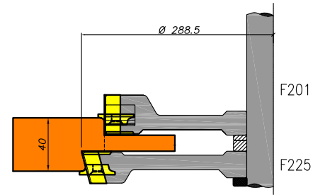
Enkele pen deuren 40mm
