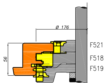
Draaikiep opdek onderdorpel
