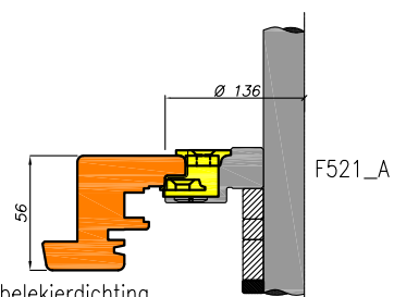
Draaikiep opdek 15mm stomp met dubbelekiërdichting
