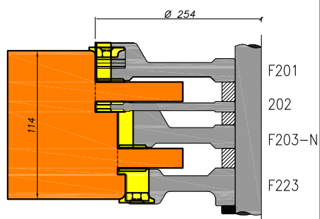
Onderdorpel
