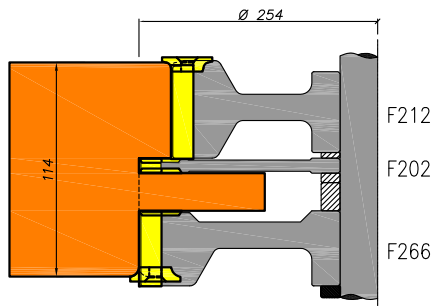
Bovendorpel / stijl
