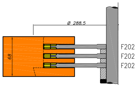
Pennen ramen 3 vlaks
