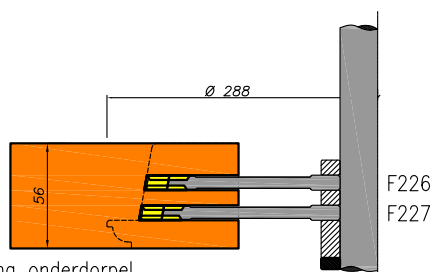
Slissen ramen buitenbeglazing onderdorpel
