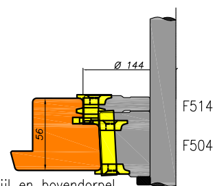
Ramen met kaderdichting en turbohol stijl en bovendorpel
