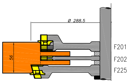
Ramen met kaderdichting stijl en bovendorpel
