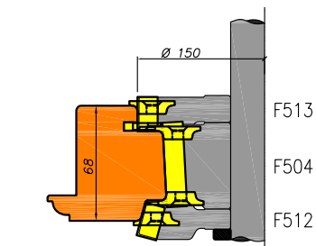
Ramen stijl en bovendorpel met kaderdichting verjongd
