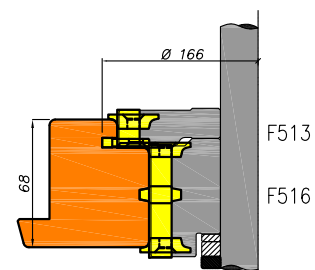
Ramen met kaderdichting onderdorpel
