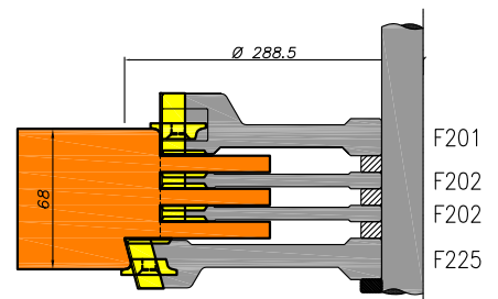
Pennen ramen 3 vlaks
