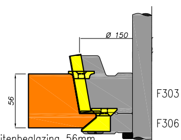
Raam-deurprofilering onderdorpel buitenbeglazing 56mm
