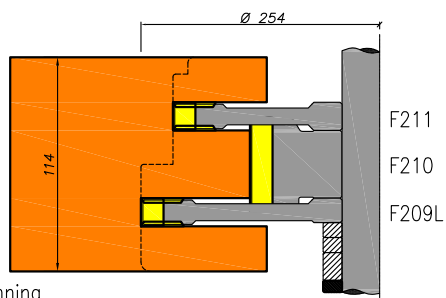
Raamprofilering / Deurprofilering
