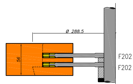
Draaikiep Contura onderdorpel
