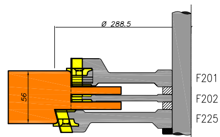
Ramen met kaderdichting stijl en bovendorpel
