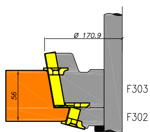
Slissen ramen buitenbeglazing
