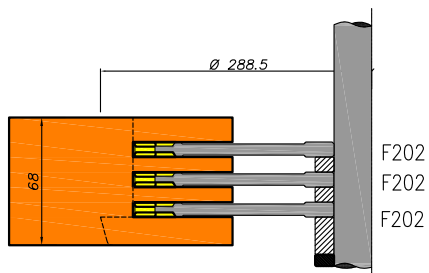
Slissen ramen 3 vlaks
