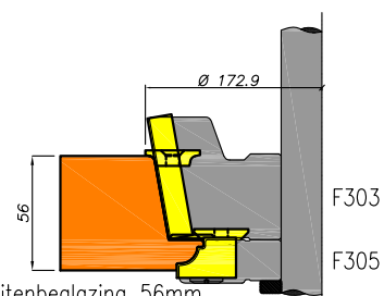
Raam-deurprofilering onderdorpel buitenbeglazing 56mm
