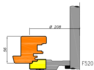
Draaikiep Contura onderdorpel
