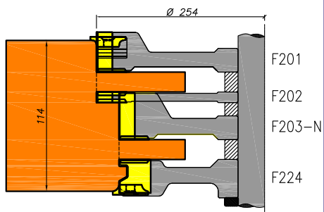
Stijl met scharniersponning
