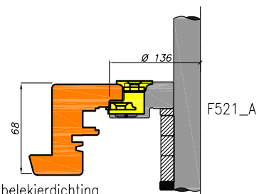
Draaikiep opdek 17mm stomp met dubbelekiërdichting
