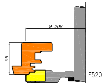
Draaikiep opdek 15mm onderdorpel
