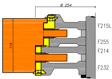
Onderdorpel
