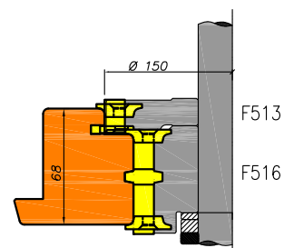
Ramen met kaderdichting onderdorpel
