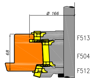
Ramen stijl en bovendorpel met kaderdichting verjongd
