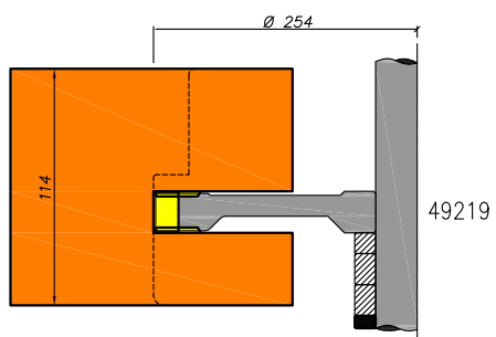
Tussendorpel / kalf - stijl
