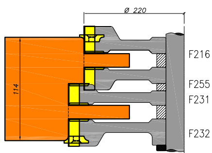
Onderdorpel
