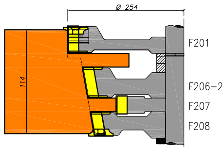
Bovendorpel met waterhol
