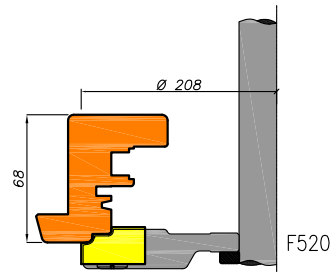
Draaikiep opdek 17mm onderdorpel
